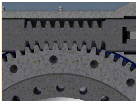
Direktantrieb mit Schneckenwelle
